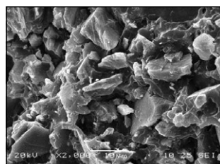
Рис. 7. РЭМ (увеличение x2000). Отвержденный силер без воздействия ЭМП. Виэдент (ВладМиВа, Россия)
