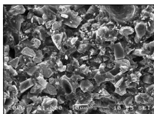
Рис. 5. РЭМ (увеличение x1000). Отвержденный силер без воздействия ЭМП. Виэдент (ВладМиВа, Россия)
