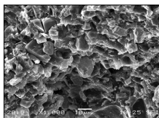
Рис. 6. РЭМ (увеличение x1000). Отвержденный силер после воздействия ЭМП. Виэдент (ВладМиВа, Россия)
