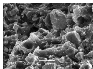
Рис. 8. РЭМ (увеличение x2000). Отвержденный силер после воздействия ЭМП. Виэдент (ВладМиВа, Россия)
