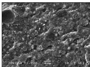
Рис. 1. РЭМ (увеличение x1000). Отвержденный силер без воздействия ЭМП. Эпоксидин (Techno Dent, Россия)
